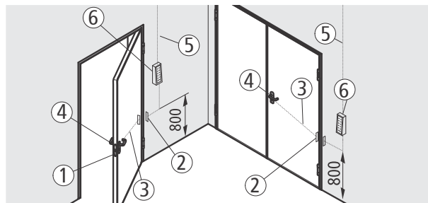
Schema componenti
